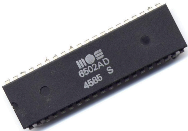
Fig. 1 - Microprocessore 6502
