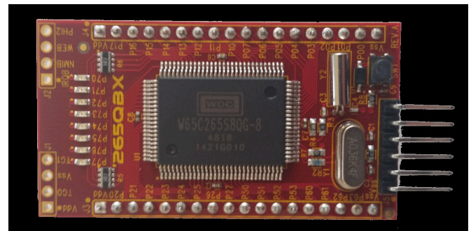
Fig. 5 - Il microcomputer MENSCH™ (codice W65C265QBX) è un piccolo computer a scheda singola (SBC), 1,25" x2.25", che utilizza il System on a Chip (SoC) W65C265S MCU, inventato e progettato da Bill Mensch.
