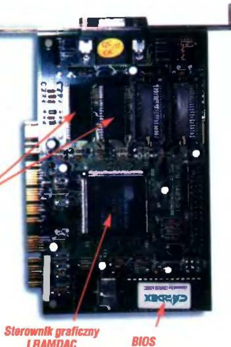
Rys. 2. Karta graficzna starszego typu
