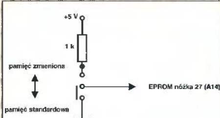
Fys. 2. Schemat przełącznika bloków pamięci
