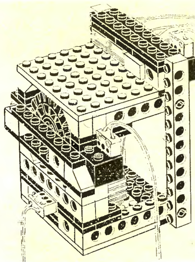
Rys. 1 Model pralki automatycznej z klocków LEGO
