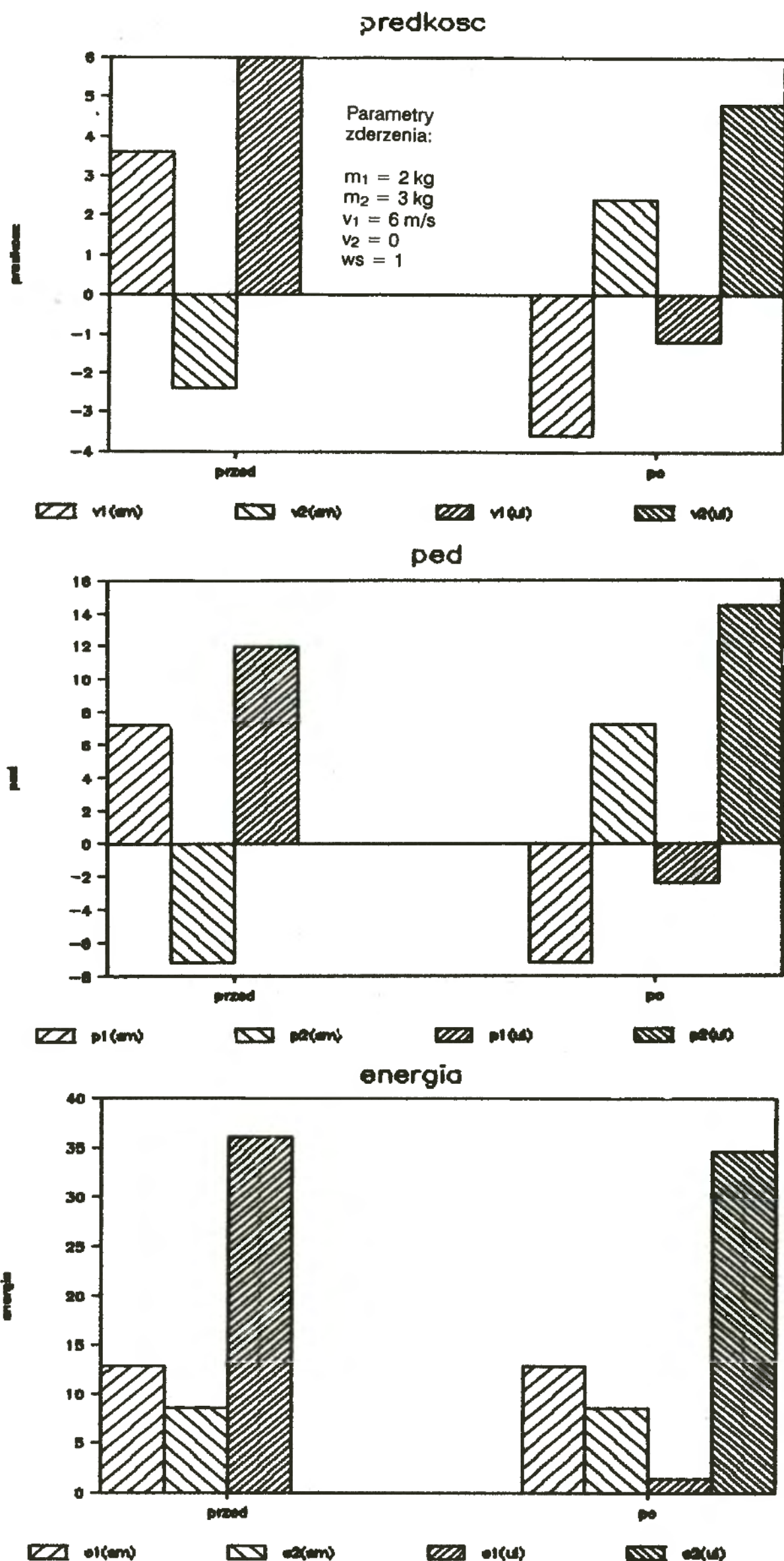
Rys. 5 Zderzenie sprężyste. Bilans prędkości, pędu i energii
