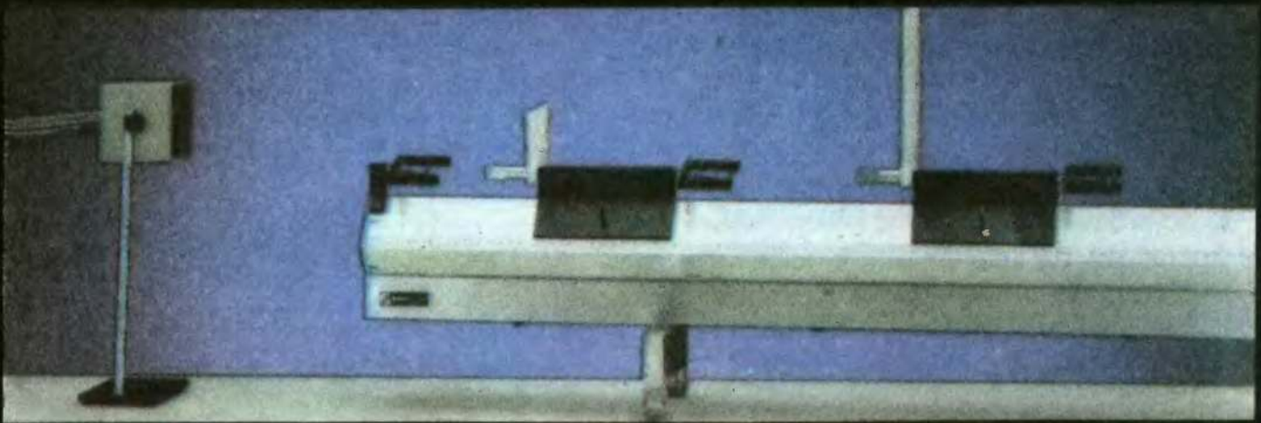
Zderzenia na torze powietrznym: a) zestaw pomiarowy b) wykres położenia c) wykres prędkości
