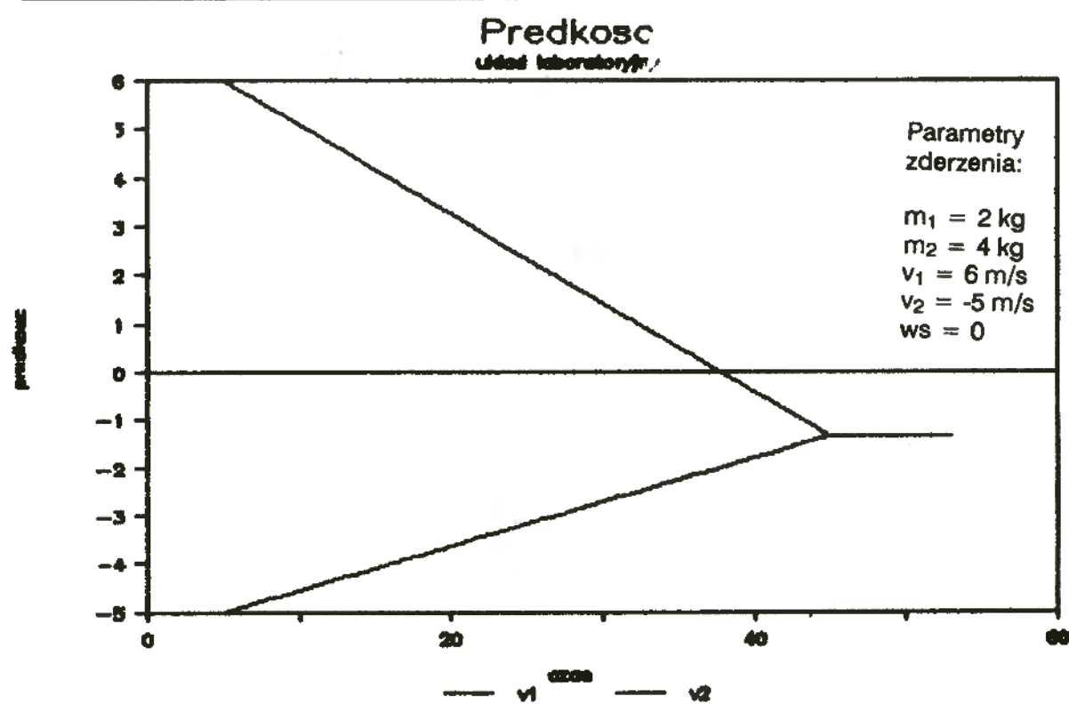
Rys. 2 Zderzenie sprężyste — układ laboratoryjny
