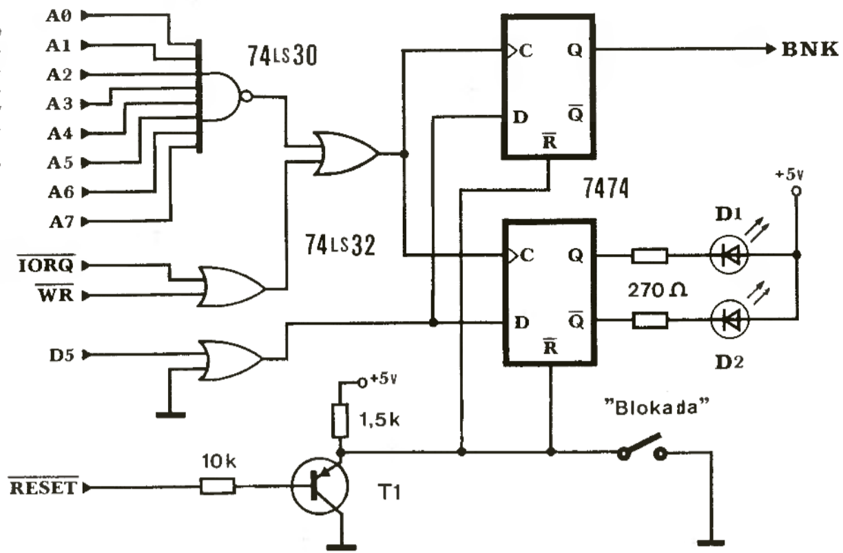
Rys. 1 Schemat układu przełączania banków
