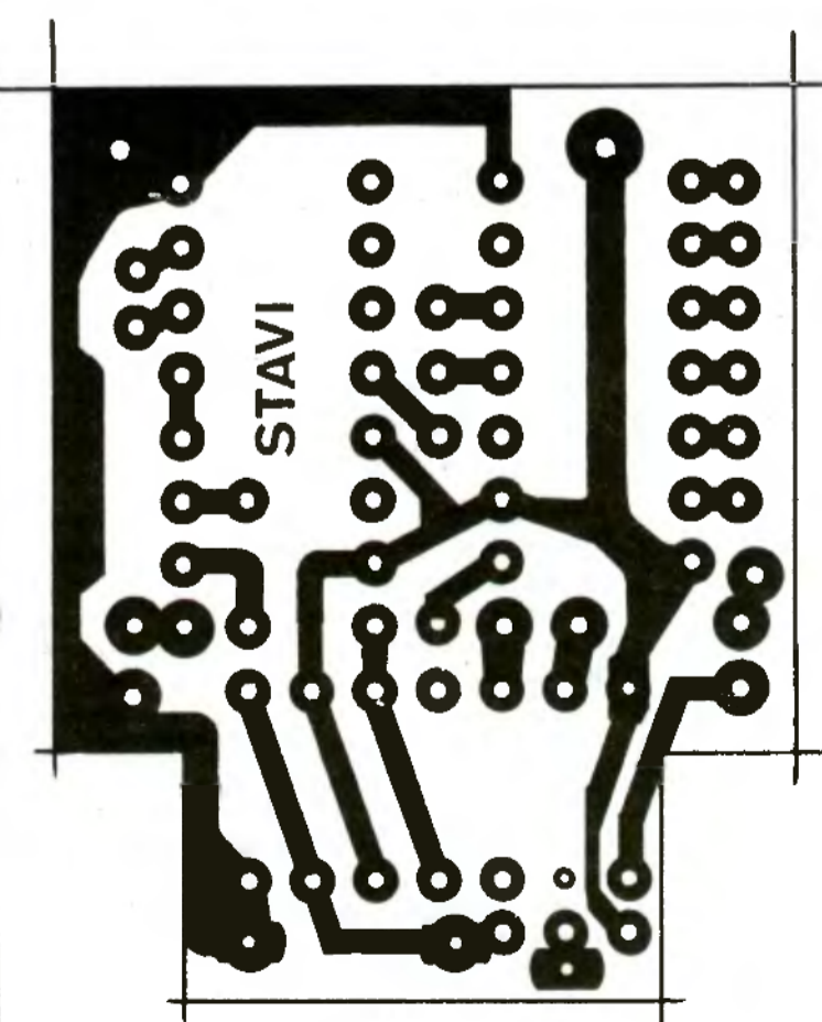
Rys. 2a Rysunek płytki drukowanej
