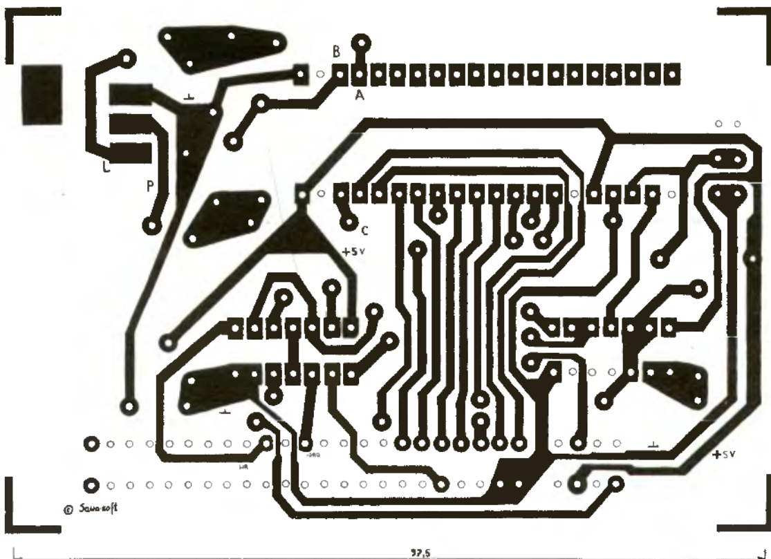
Rys. 2 Widok płytki do AY-3-8910 SOUND INTERFACE
