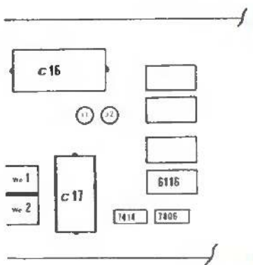
Rys. 1. Lokalizacja złączy J1 i J2 na płycie.
