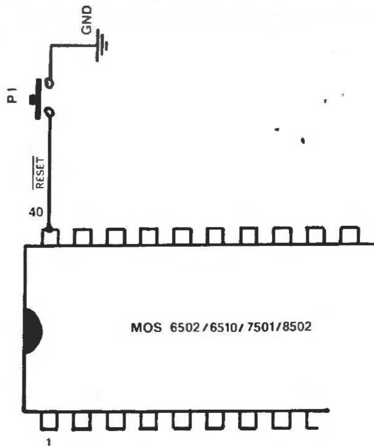
RYSUNEK 1 — Zasada działania przycisku RESET — wolny przełącznik astabilny (może być nawet wykonany z małego isostatu), dwa długie izolowane przewody (najlepiej linka), lutownica o mocy do 25 W, cyna i kalafonia.
