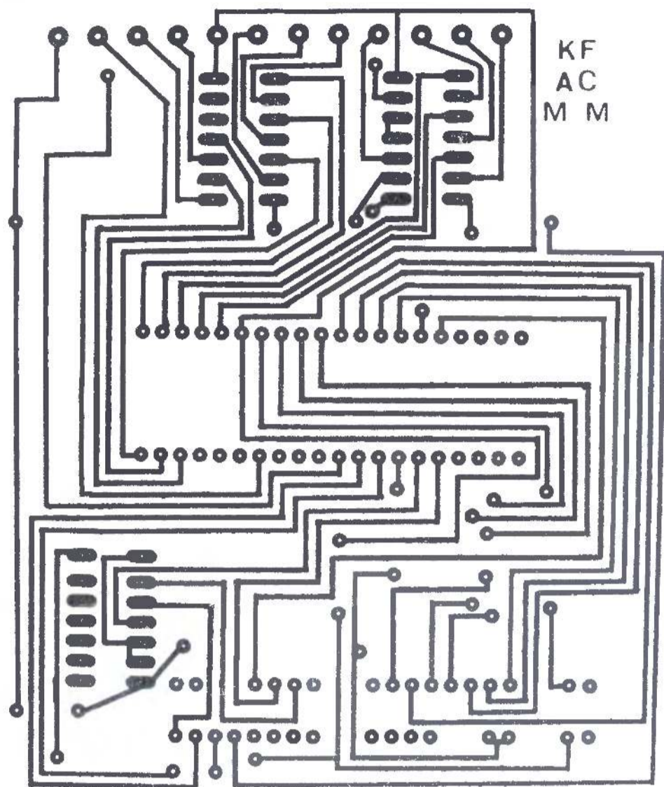
Rys. 2 Płytkę drukowaną interfejsu skala 1:1
