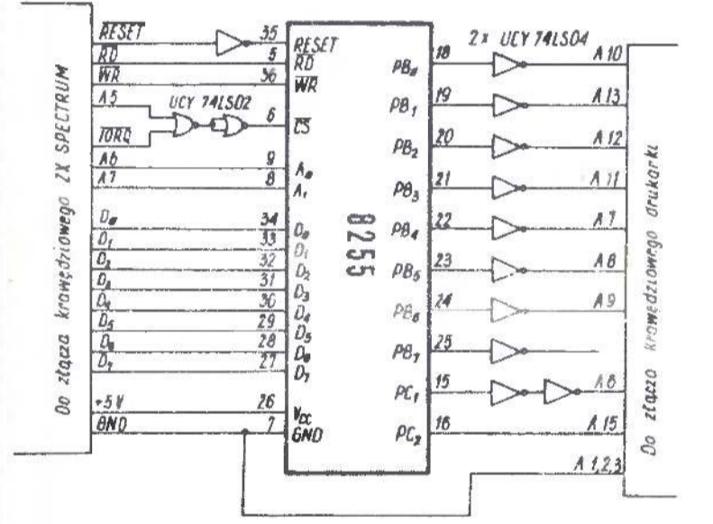
Rys. 1 Schemat ideowy interface'u
