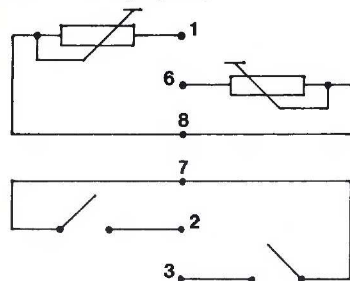
Rys. 2. Schemat elektryczny zespołu wioselki.
