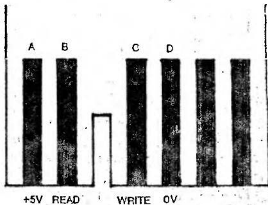
Rys. 2. Widok szyny kontaktowej od strony druku
