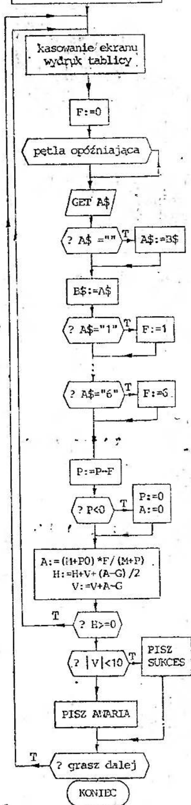
Schemat blokowy algorytmu
