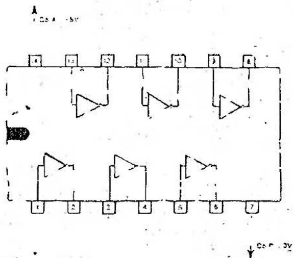
Rys. 1. Schemat wyprowadzeń układu UCY 7404 (widok z góry)
