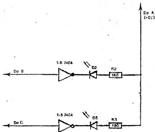
Rys. 3. Schemat ideowy sygnalizatora
