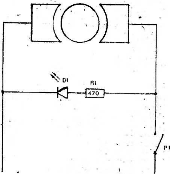
Rys. 4. Schemat podłączenia diody sygnalizującej pracę silnika
