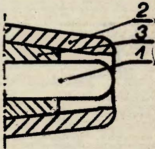
Rys. 5. Sposób zamocowania fototranzystora. 1 — fototranzystor, 2 — obudowa, 3 — podkładka gumowa.
