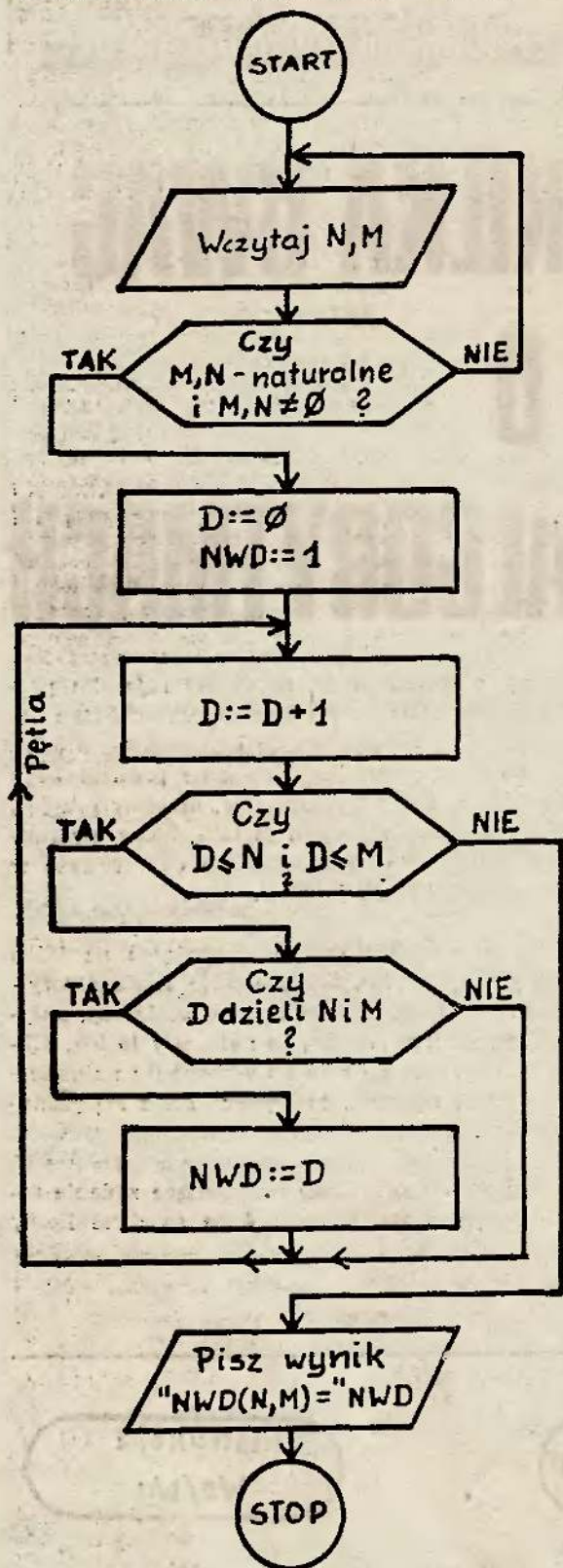
Rys. 2. Schemat blokowy algorytmu „siłowego” znajdowania NWD dwóch liczb naturalnych
